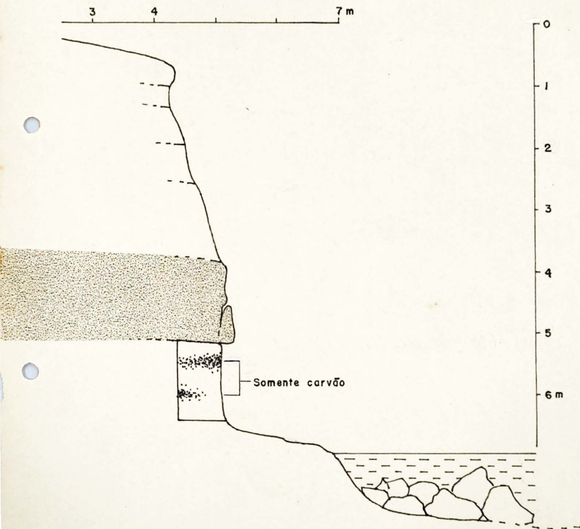
SITIO RS-1-72: PALMITO-2. Corte Estratigráfico e Níveis Arqueológicos
